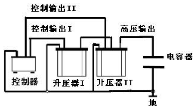
图 11 测量电容器的连线图
