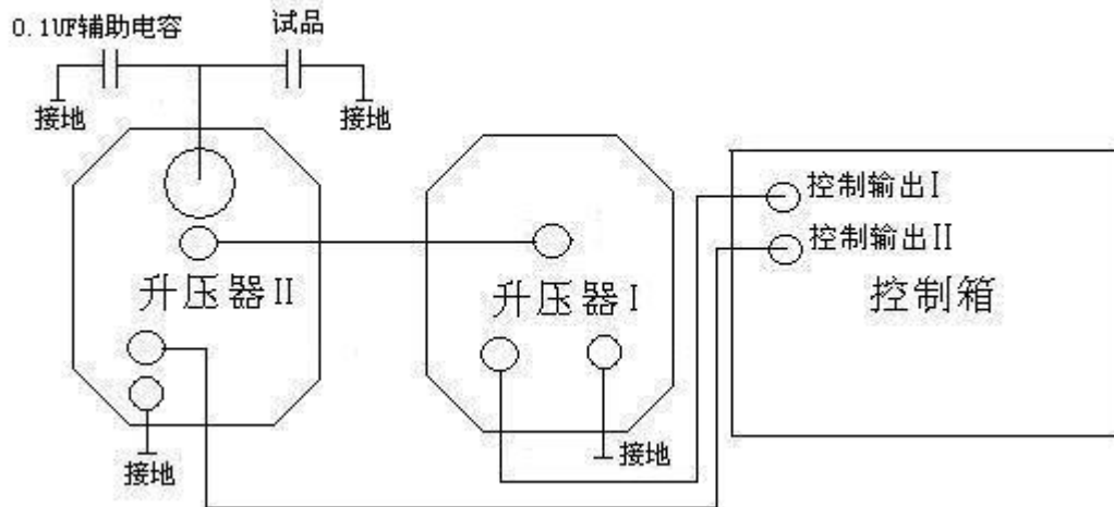
图 4 （连线图）
