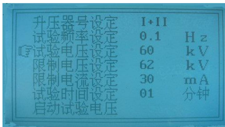
图 5（设定界面）
